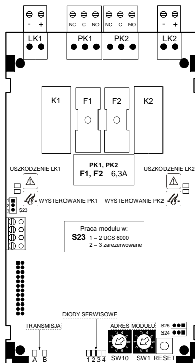
Rys. 4.4 Moduł MPW-60
