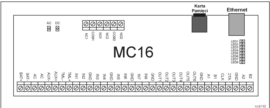
Rys. 3 Widok płyty MC16 Tabela 1: Opis zacisków
