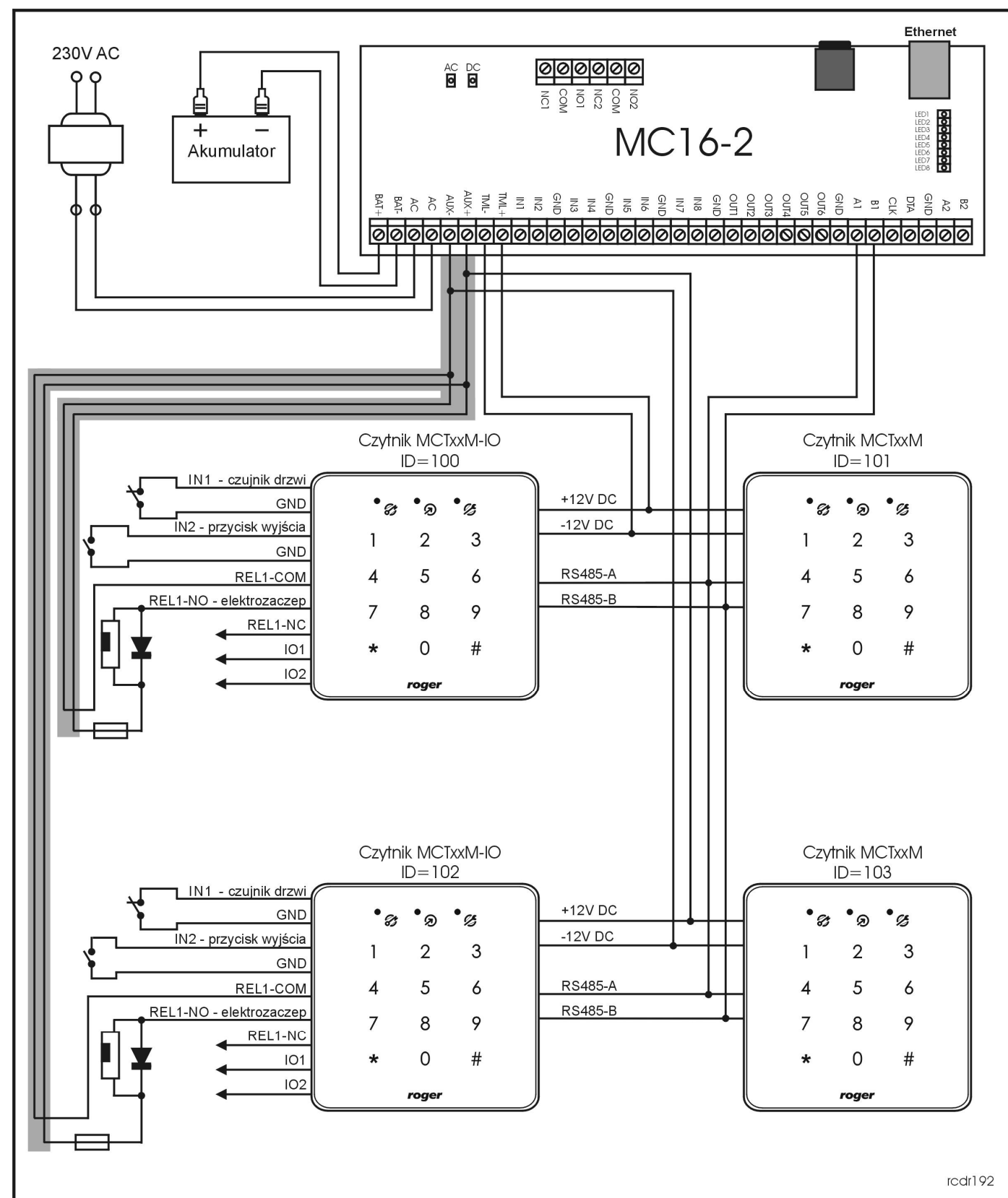
Rys. 9 Przykład realizacji kontroli dostępu dla dwóch przejść obustronnie kontrolowanych zasilanych z wbudowanego zasilacza MC16.
