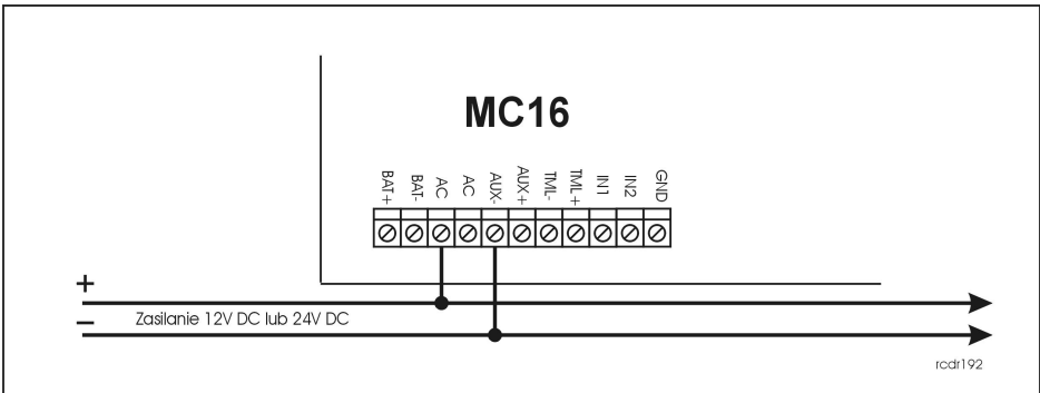
Rys. 2 Sposób podłączenia zasilania napięciem DC.
