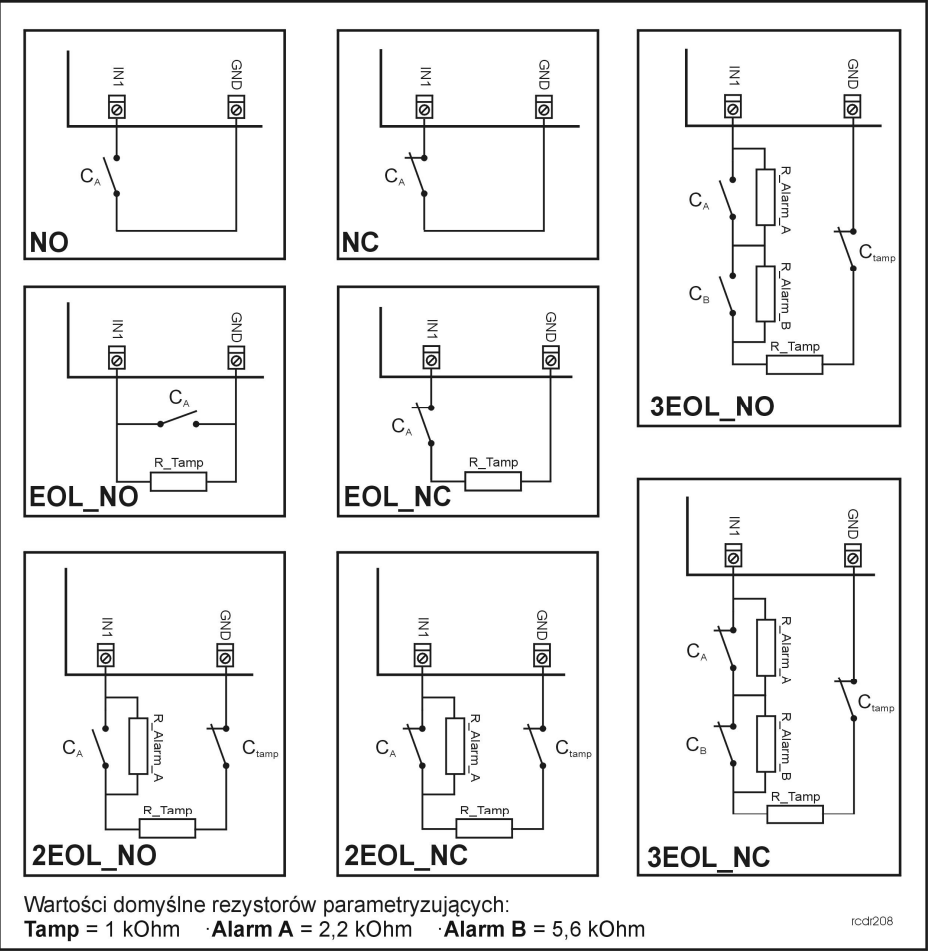
Rys. 6 Topologia wejść parametrycznych.
