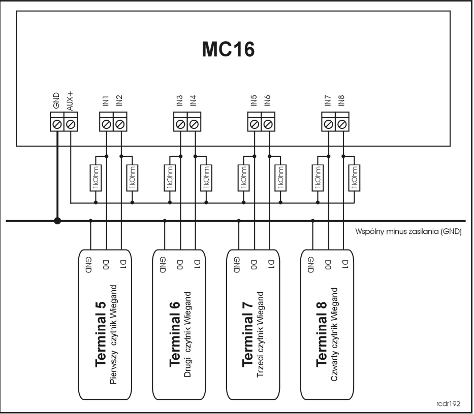
Rys. 5 Sposób podłączenia czytników Wiegand.
