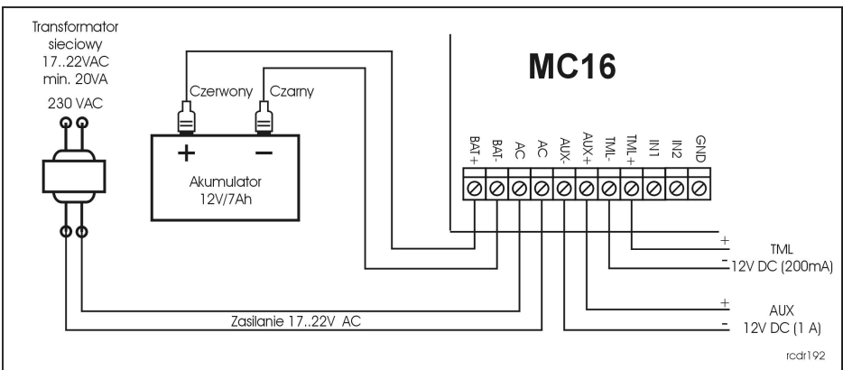
Rys. 1 Sposób podłączenia zasilania napięciem AC.
