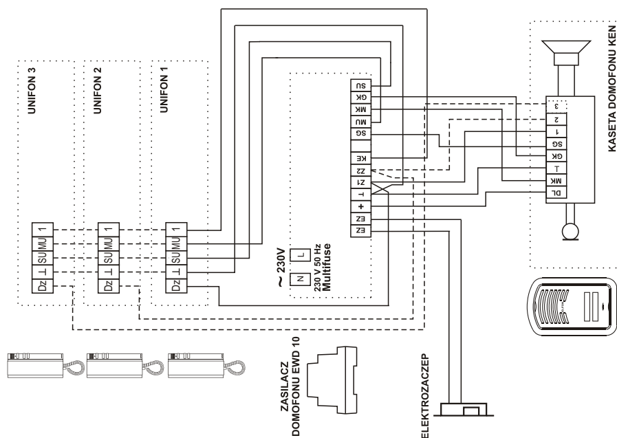
Schemat połączeń zestawu serii Z z unifonem A-U1
