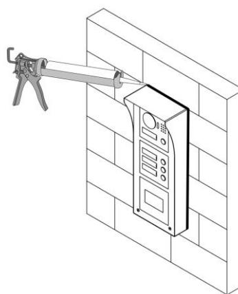
Montaż natynkowy
