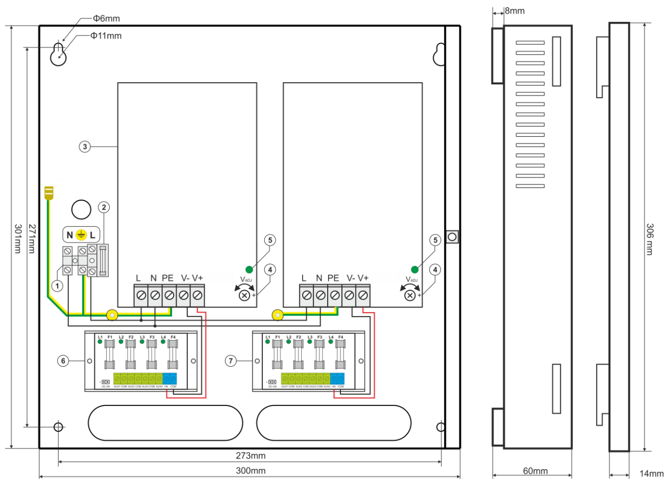
Rys.3. Widok zasilacza.
