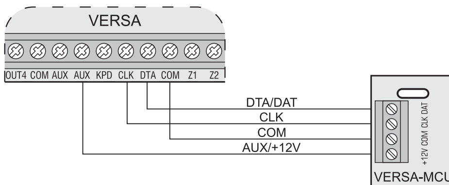
Rys. 15. Sposób podłączenia kontrolera VERSA-MCU.
