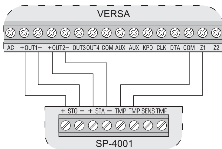
Rys. 28. Sposób podłączenia do centrali sygnalizatora bez własnego zasilania (na przykładzie SP-4001).
