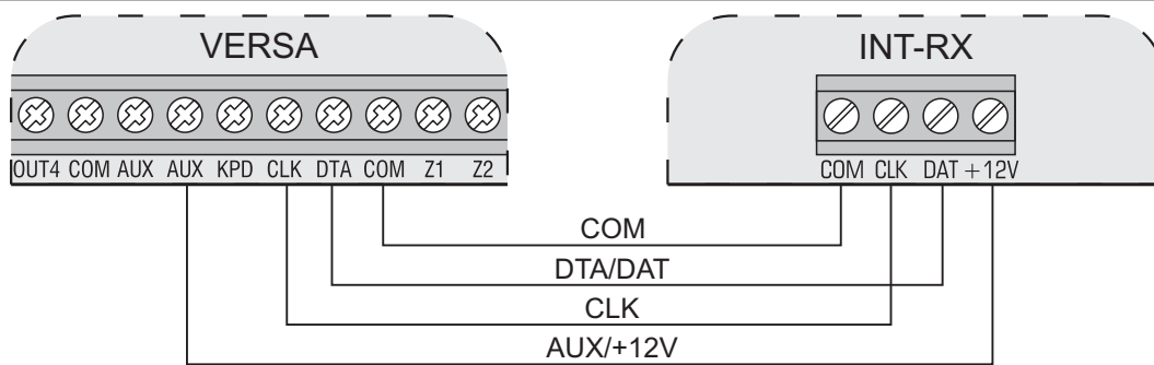
Rys. 14. Sposób podłączenia ekspandera INT-RX.
