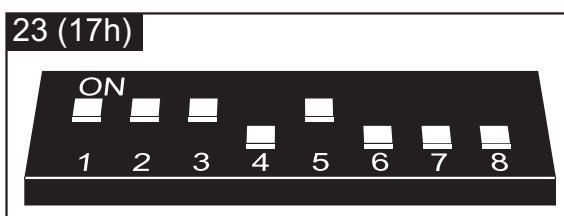
Rys. 23. Sposób ustawienia adresu w ekspanderze CA-64 SM lub module INT-VG. Ósmy przełącznik jest w pozycji OFF, czyli funkcja nagrywania komunikatów głosowych jest zablokowana.
