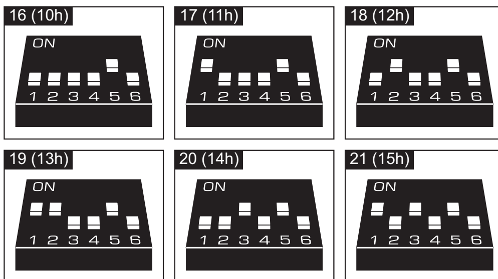
Rys. 22. Sposób ustawienia adresów na przykładzie modułu INT-IT.
