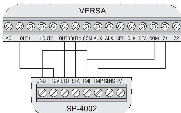
Rys. 29. Sposób podłączenia do centrali sygnalizatora z własnym zasilaniem (na przykładzie SP-4002). Dla wyjść OUT3 i OUT4 należy zaprogramować odwrotną polaryzację. Kołki PLO i PLA w sygnalizatorze muszą być rozwarte (sygnalizacja wyzwalana po odcięciu masy).
