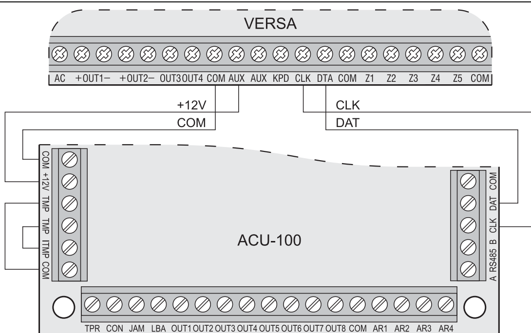
Rys. 17. Sposób podłączenia kontrolera ACU-100. Zaciski TMP styku sabotażowego kontrolera podłączone są do obwodu sabotażowego kontrolera (zaciski ITMP i COM), dzięki czemu informacja o naruszeniu styku sabotażowego kontrolera przekazywana jest do centrali za pośrednictwem magistrali komunikacyjnej. Jeżeli zaciski TMP nie są podłączone do obwodu sabotażowego kontrolera, zacisk ITMP należy zewrzeć do masy.
