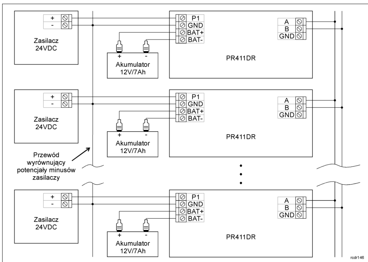
Rys. 7 Zasilanie kontrolerów PR411DR napięciem 24VDC
