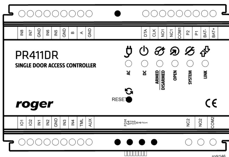
Rys. 1 Kontroler PR411DR
