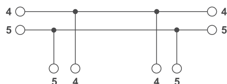
Schemat połączeń 2
