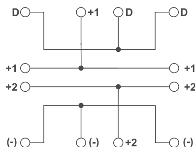
PIP-3AN/Rozgałęźna
