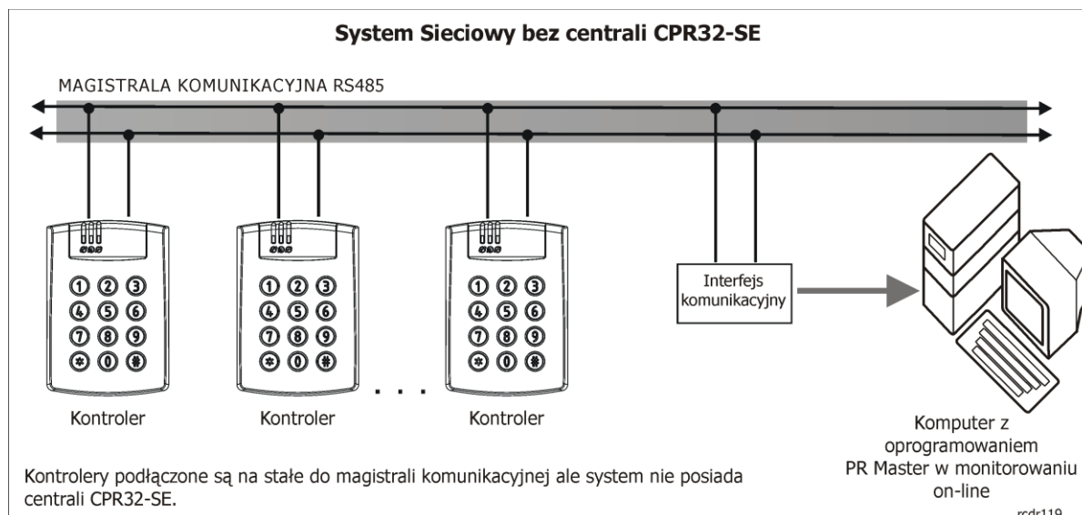
Rys. 5 Praca w Trybie Sieciowym (bez centrali CPR32-SE)
