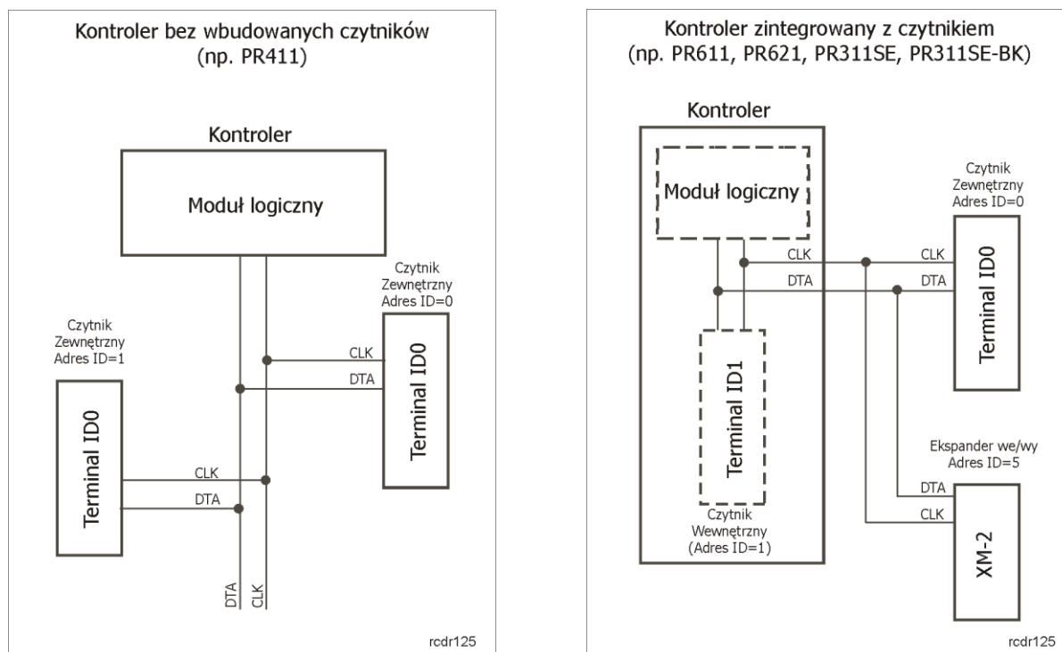
Rys. 6 Interfejs RACS Clock&amp;Data
