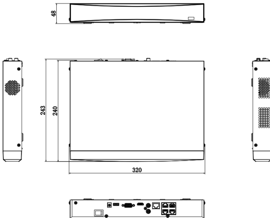
scale/1:1;Unit/mm
