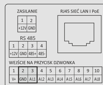
Terminal przyłączeniowy
