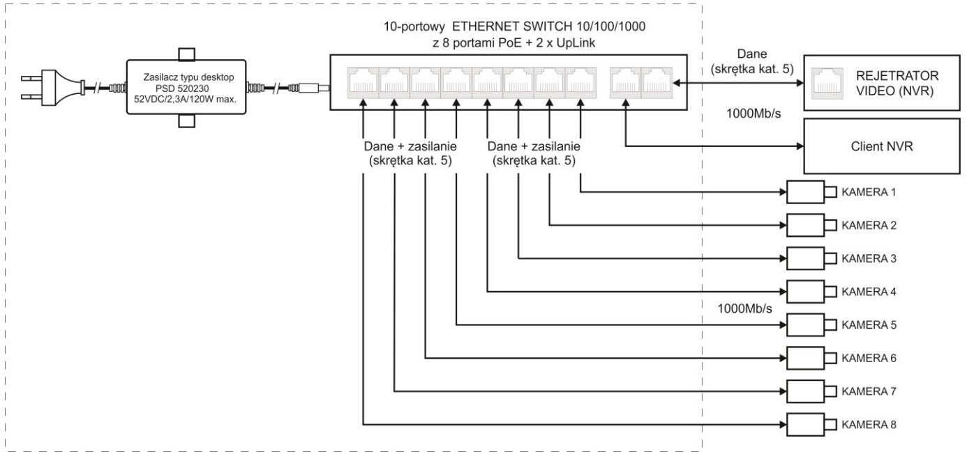
Rys. 1. Schemat blokowy.
