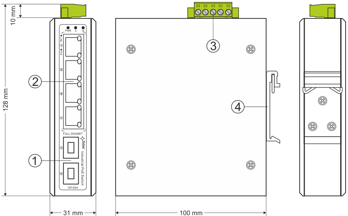
Rys. 2. Widok switch'a.
