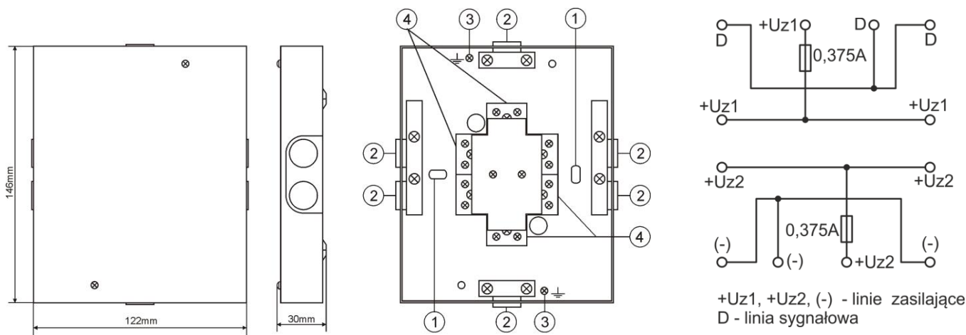
Rys.1. Widok puszek instalacyjnych i schemat połączeń.
