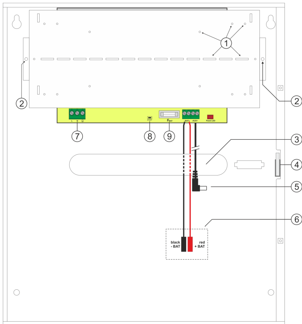
Rys.3. Widok zasilacza.
