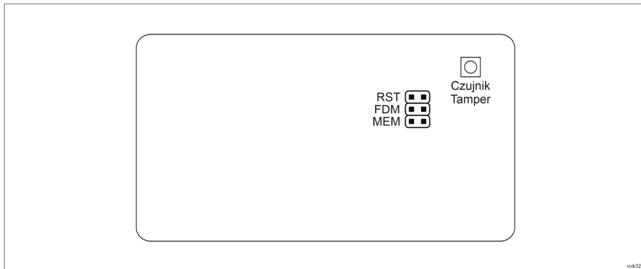
Rys. 4 Zworki programujące
