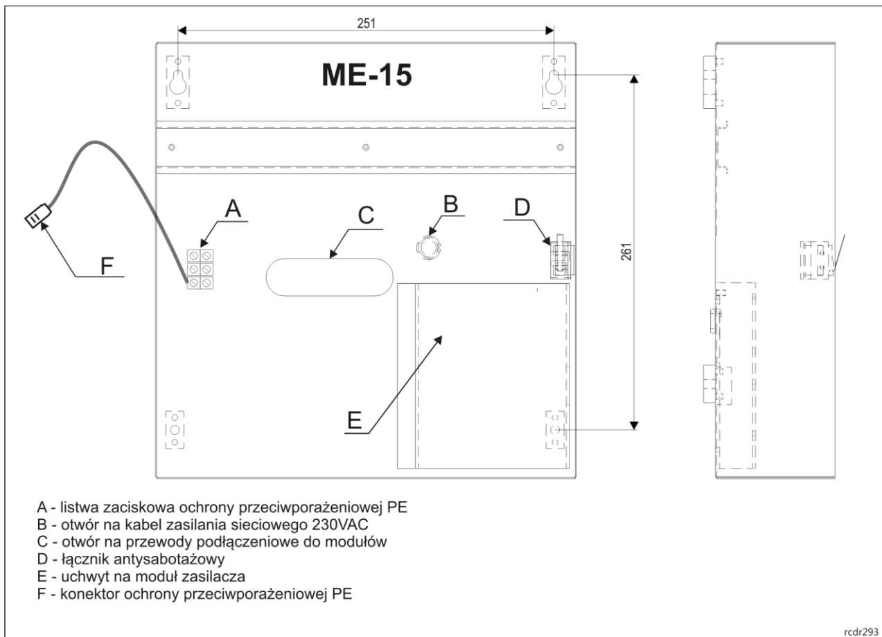
Rys. 1 Widok wnętrza obudowy ME-15
