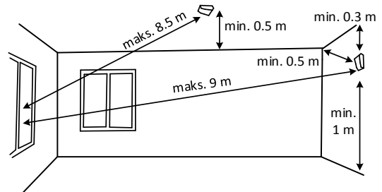
Położenie detektora przy instalacji na ścianie lub suficie
