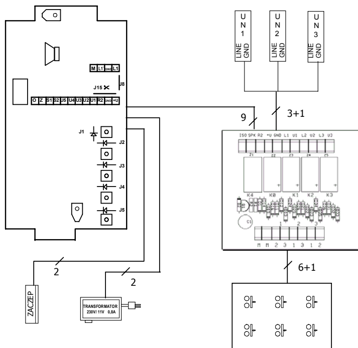
Rys. 2 Schemat blokowy podłączenia modułu interkomu.
