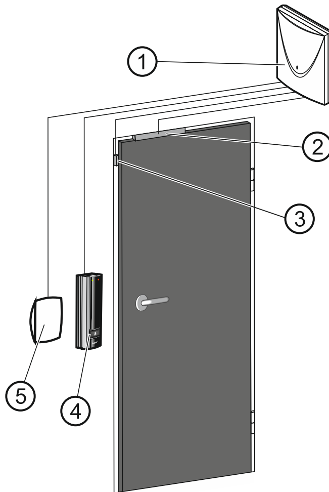
Rys. 8. Przykładowa instalacja kontroli dostępu.
