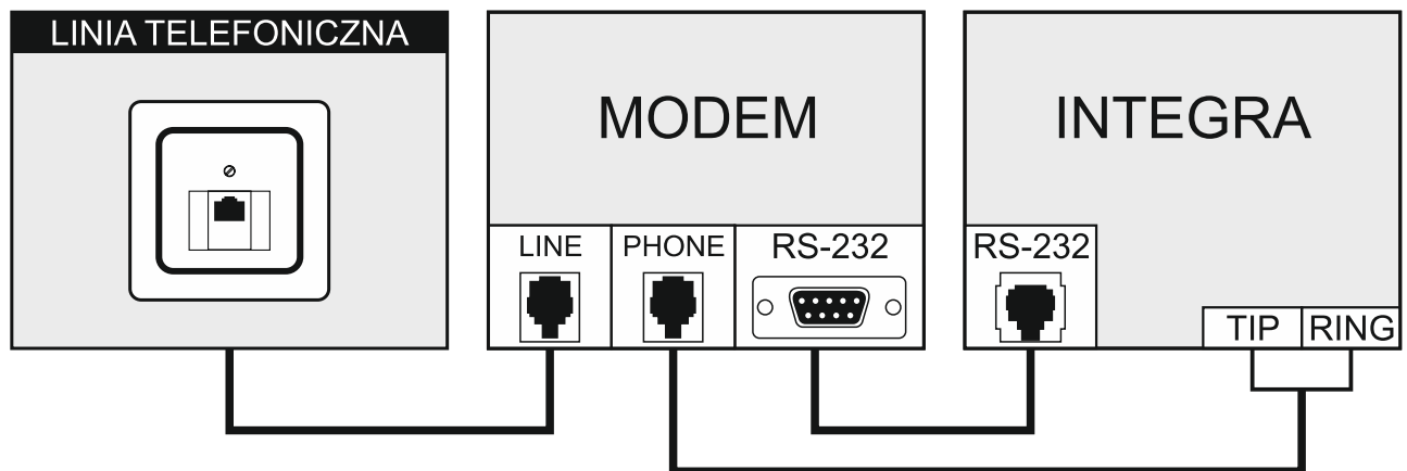
Rys. 14. Schemat podłączenia analogowego modemu zewnętrznego do centrali.
