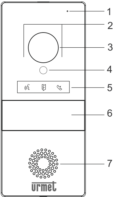
Widok przód
