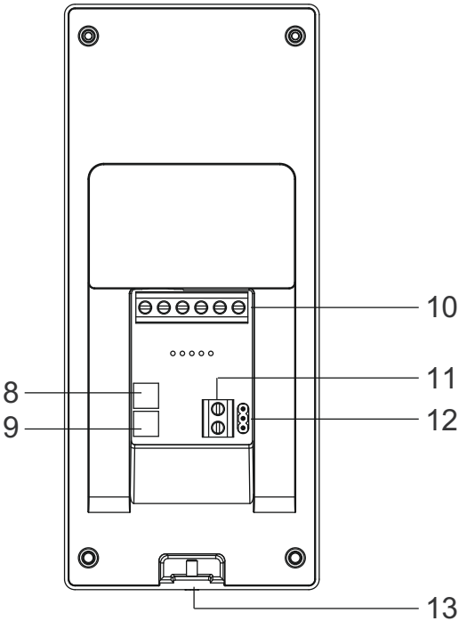
Widok tył
