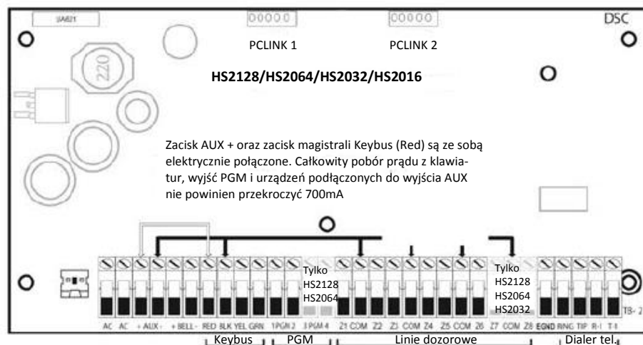
Rysunek 2-1 Prowadzenie przewodów
