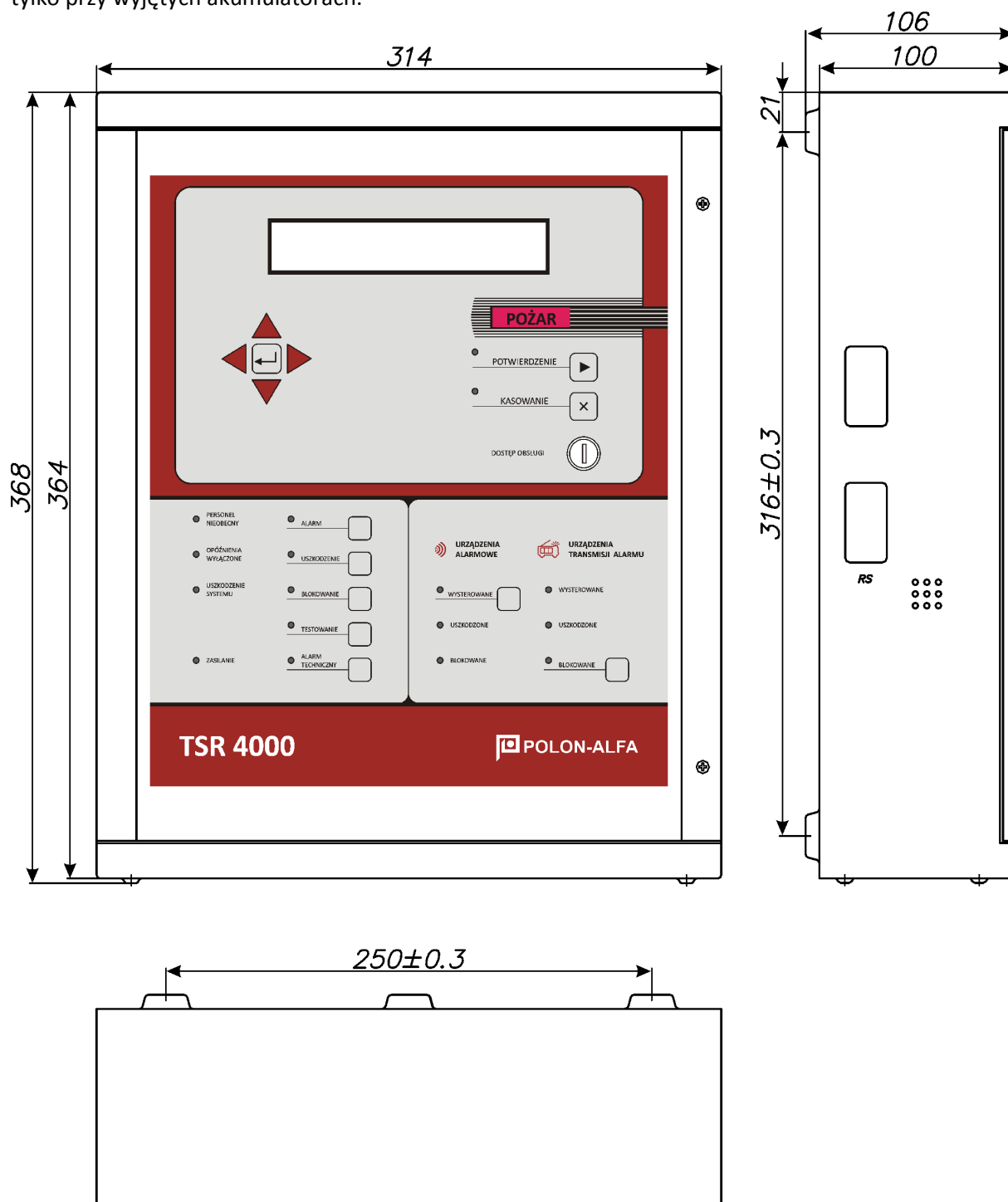
Rys. 7.1. Widok i podstawowe wymiary terminala TSR-4000
