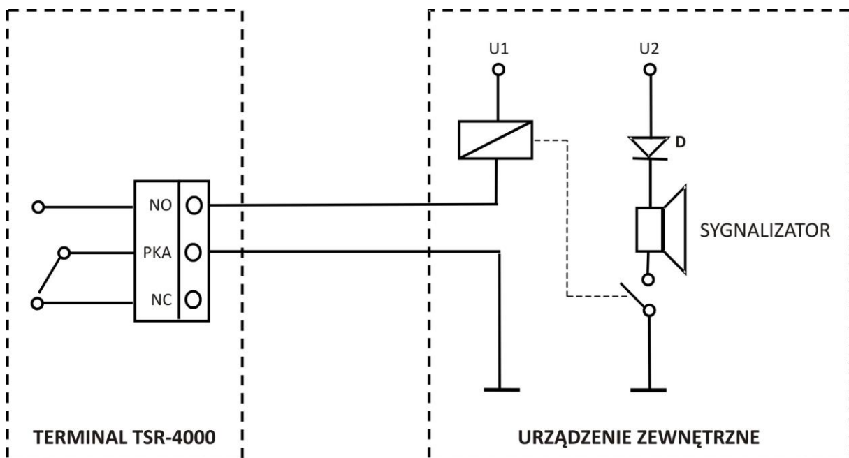
Rys. 5.8.1 Przykładowe rozwiązanie nadzorowania wyjścia przełącznikowego
