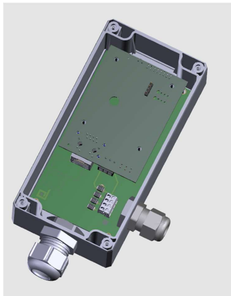
Rysunek 8.6.2 Widok ogólny modułu MKI
