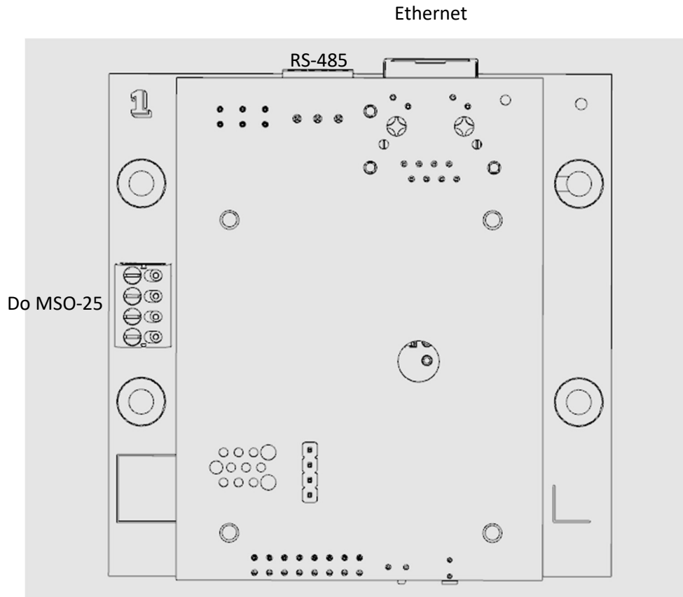
Rysunek 8.5.2 Moduł MKE-25
