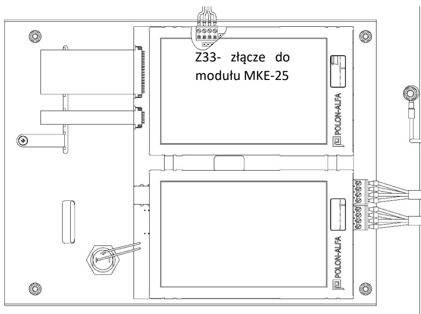
Rysunek 8.5.3 podłączenie modułu MKE-25 do modułu MSO-25
