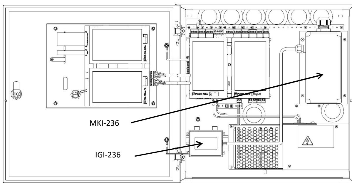
Rysunek 8.6.4 montaż modułu UIK-236 w obudowie centrali
