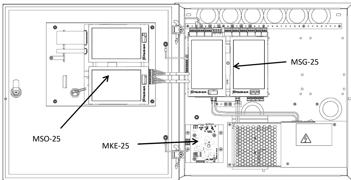
Rysunek 8.5.1 Moduł MKE-25 zamontowany w obudowie
