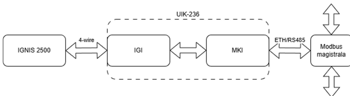
Rysunek 8.6.3 Schemat blokowy połączenia modułu z centralą IGNIS 2500
