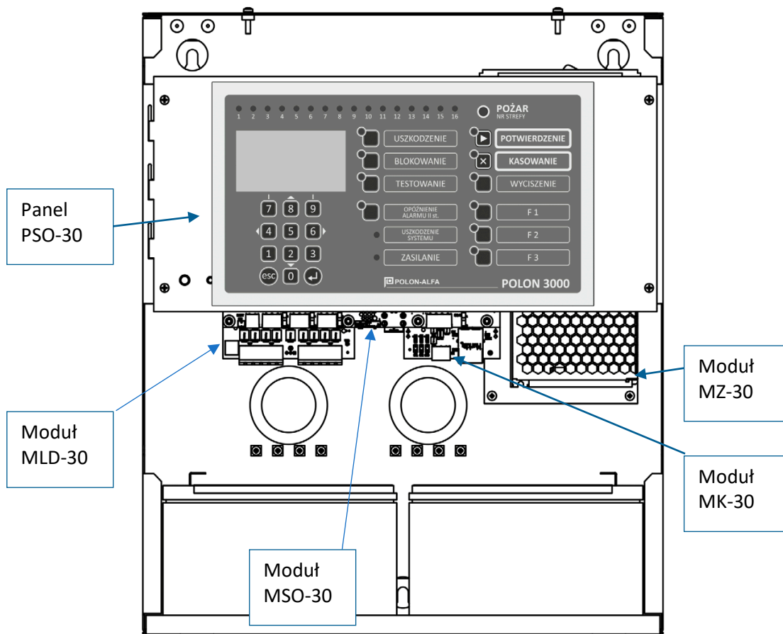
Rys. 5-2 Moduły centrali
