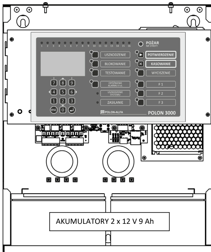
Rys. 6-2 Widok położenia akumulatorów w obudowie
