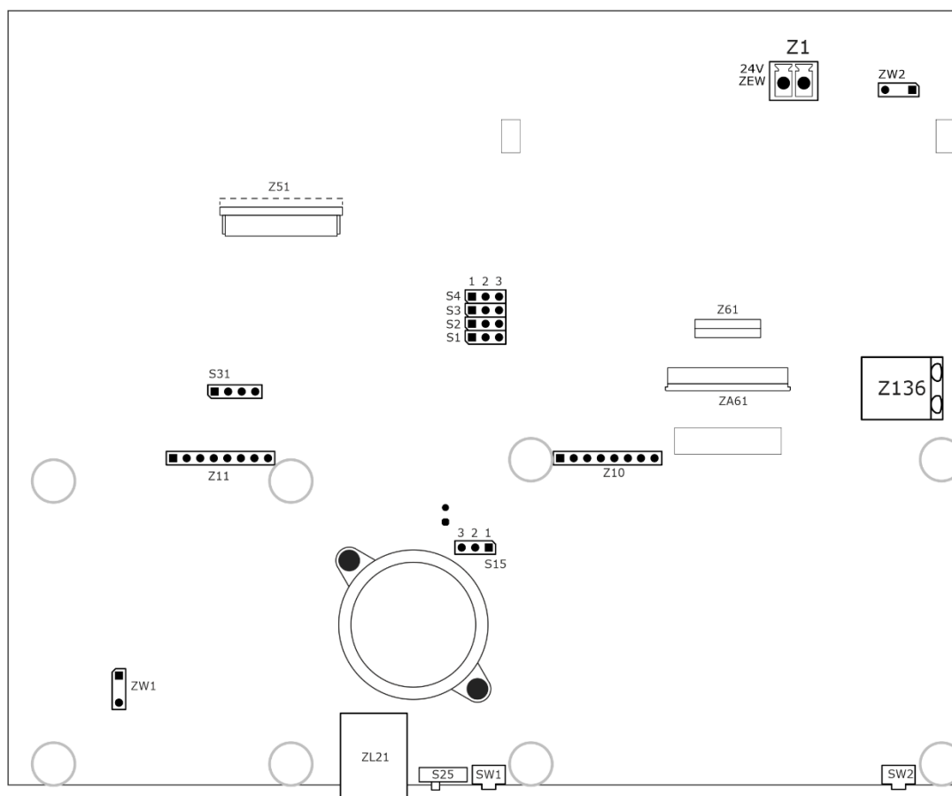
Rys. 5-5 MSO-30 - strona tylna
