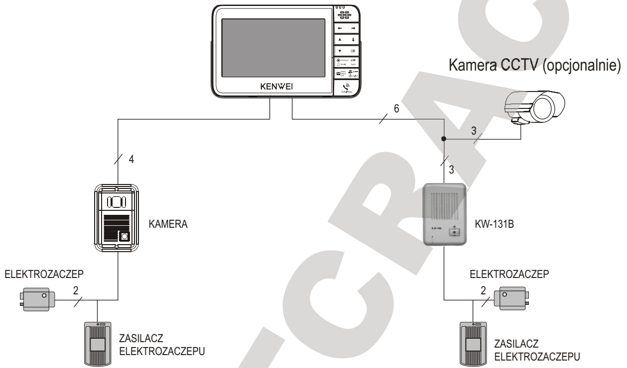
schemat modułowy
