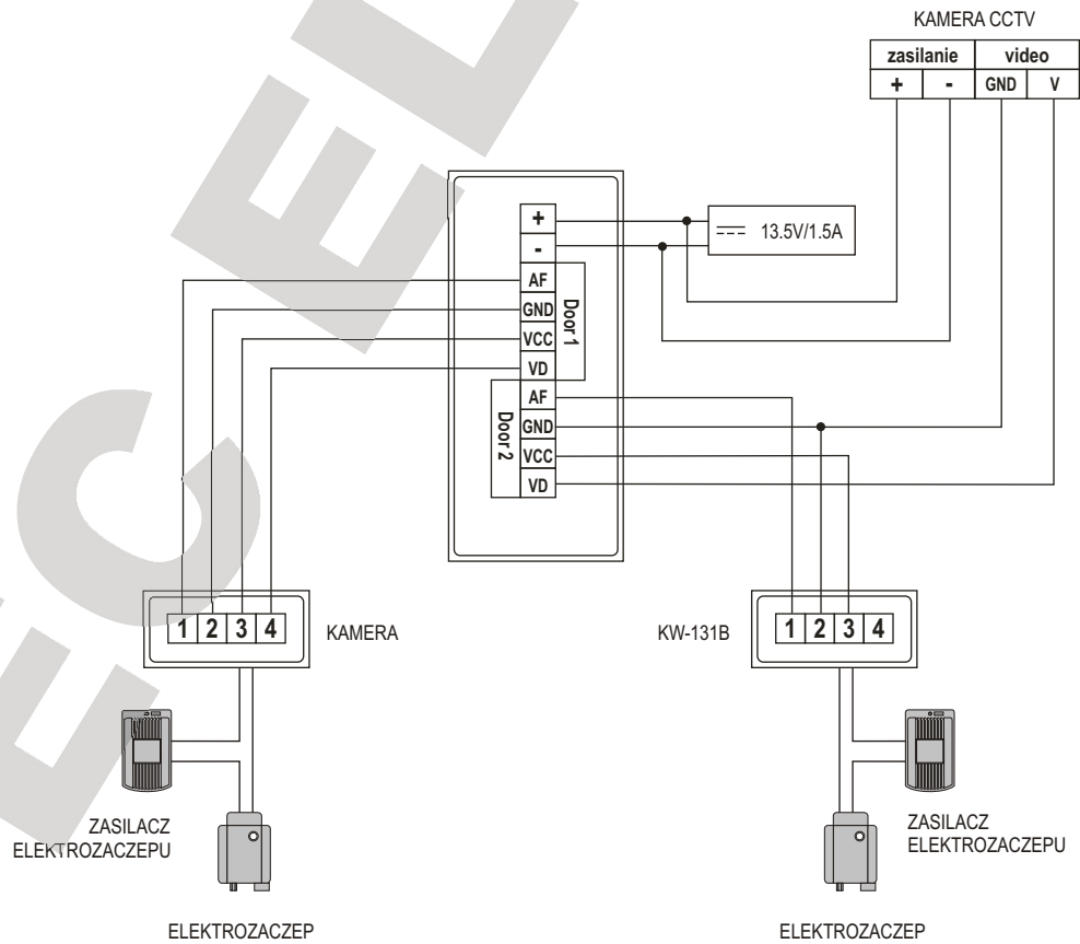
schemat podłączenia
