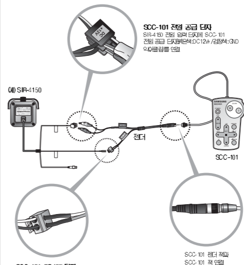
SCC-101 RS485 단자 SIR-4150 TRX(WHITE) 신호 전선 WHITE색 단자와 연결 SIR-4150 TRX(BLACK) 신호 전선 GRAY색 단자와 연결
